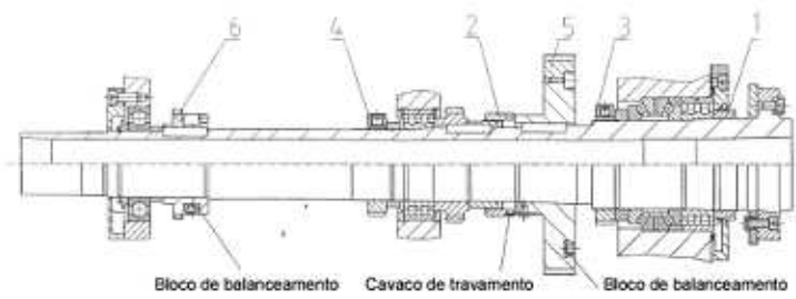
Fig. 9 Diagrama de ajuste dos mancais do fuso-mestre
