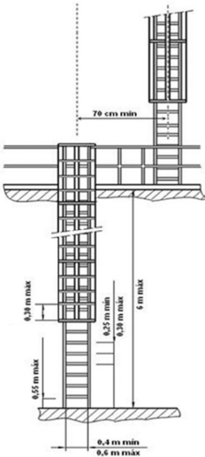
Figura 4A, 4B e 4C: Exemplo de detalhe da gaiola da escada fixa do tipo marinho.
