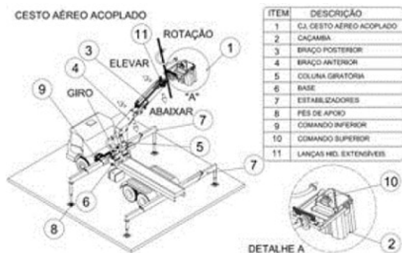
FIGURA 1: EXEMPLO DE ARRANJO COM CESTO ACOPLADO
