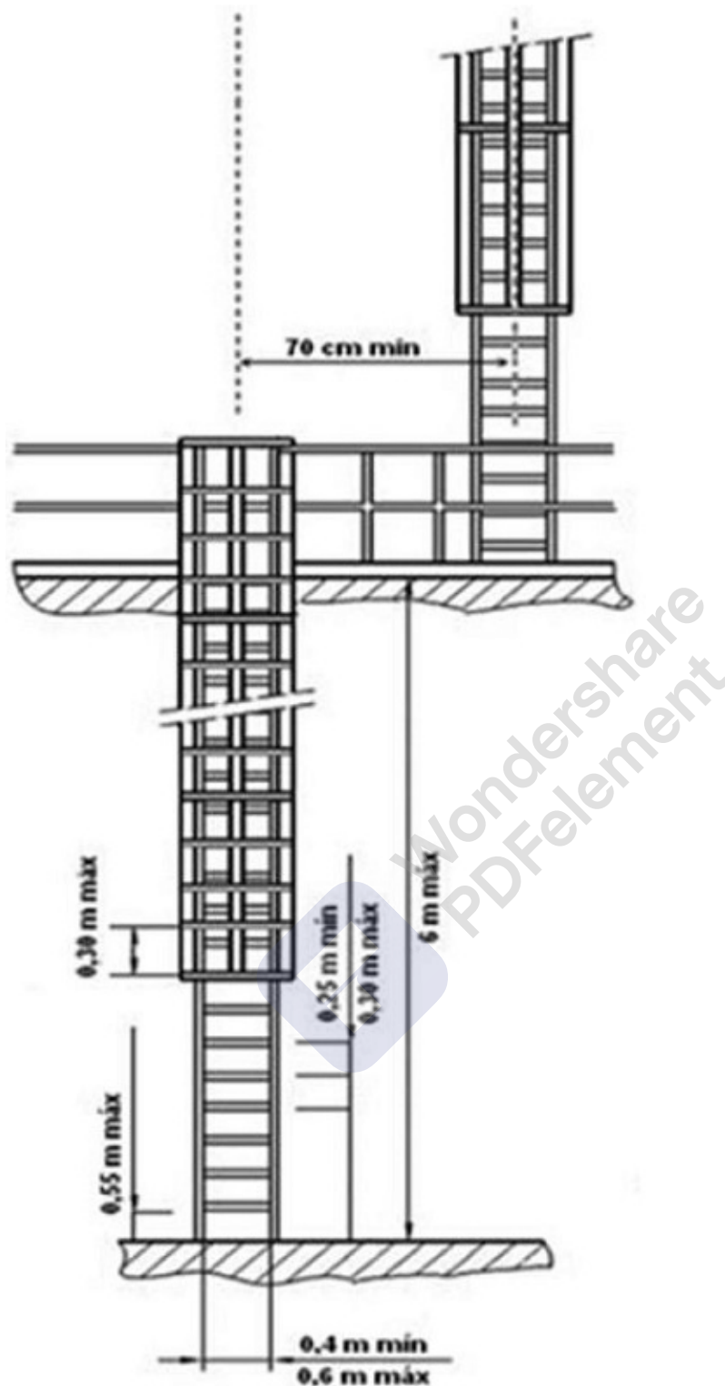
Figura 4A, 4B e 4C: Exemplo de detalhe da gaiola da escada fixa do tipo marinho.
